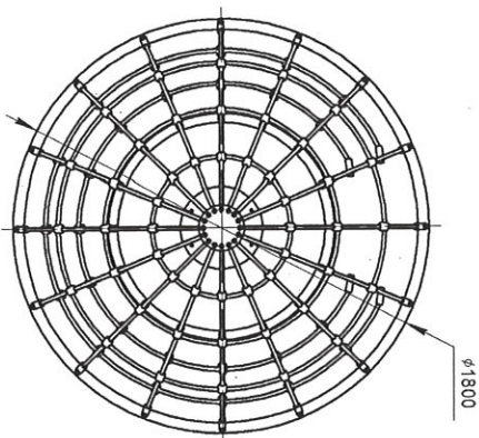
Рисунок 2 - Вид сверху
